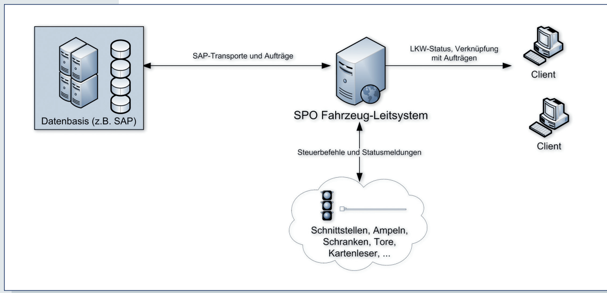
Systematische Systemarchitektur des Leitsystems zur LKW-Abwicklung
